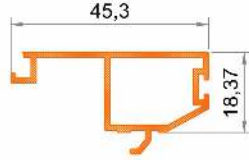
Kıl Fitilli Alüminyum Eşik Kapaması Aluminium Threshold Closing With Wick for Sliding Алюминевый порог غطاء كادر ألومنيوم بفراشي للسحاب
