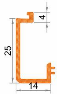
Eşik Kapama Profili Threshold Cover Profile Профиль порога بروفيل غطاء الكادر
