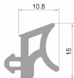
17mm cam conta Glass joint for 17 mm 17 мм уплотнитель стекла جوان للزجاج ١٧مم
