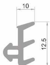
19-20mm cam conta Glass joint for 19-20 mm 19-20 мм уплотнитель стекла جوان للزجاج ١٩-٢٠مم
