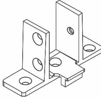
Fens 500 / ٥٠٠ Orta kayıt bağlantı takozu Mullion Fitting Wedge Закладная соединения импоста لقمة لربط بروفيل تي
