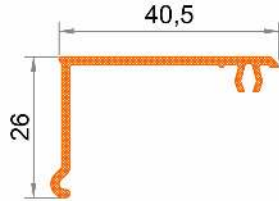
Geniş Kanal Kapama Profili Large Slot Cover Profile Широкий облицовочный профиль канала بروفيل غطاء القناة العريضة
