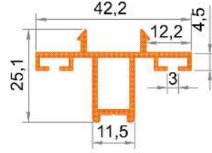
Ara Kilitleme Profili Sliding Locking Profile Профиль среднего запираения بروفيل قفل داخلي
